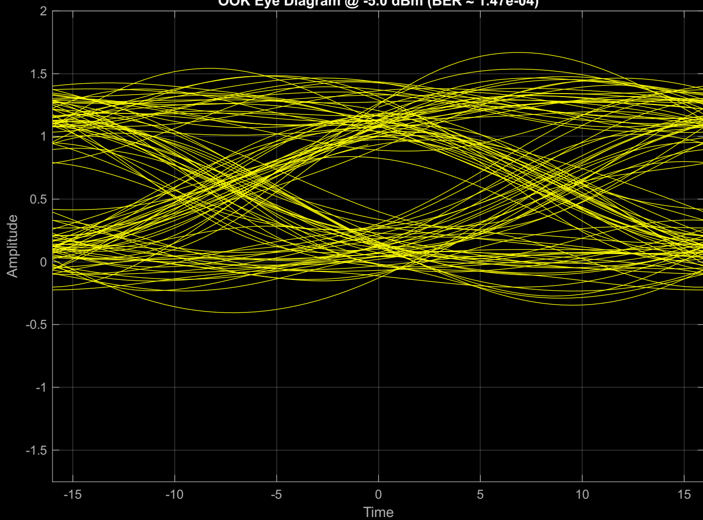
OOK Eye Diagram @ -5.0 dBm (BER \approx 1.47\text{e-}04 )
